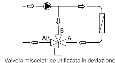
Valvola miscelatrice utilizzata in deviazione
