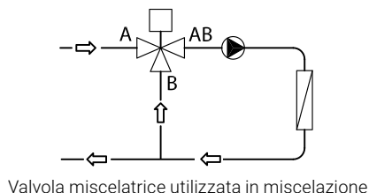
Valvola miscelatrice utilizzata in miscelazione
