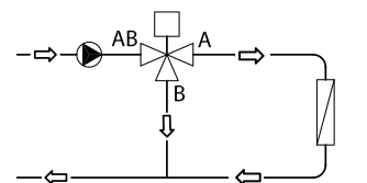
Valvola deviatrice utilizzata in deviazione
